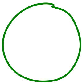
benzene
